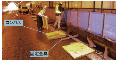
コンパネ固定金具取付
