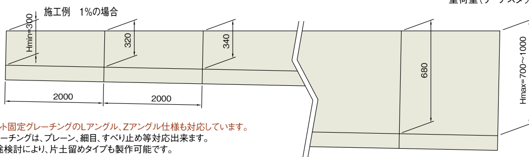
KLUグレーチング付 重荷重(リーチスタッカー)仕様
